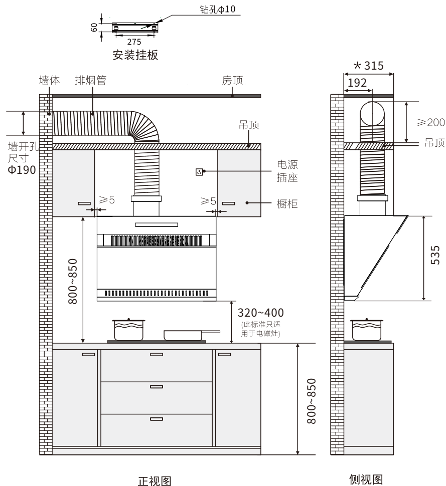
安装简图
